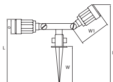
Body: PVC
